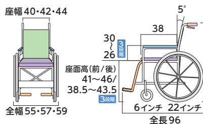
座面高モジュール 41cmと46cm比較
