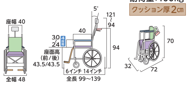
ティルト角度+5°~+30°
