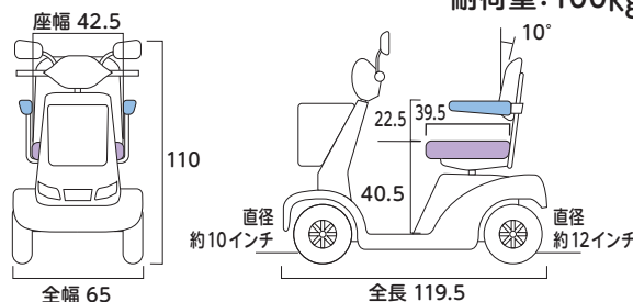
寸法図(単位:cm)
