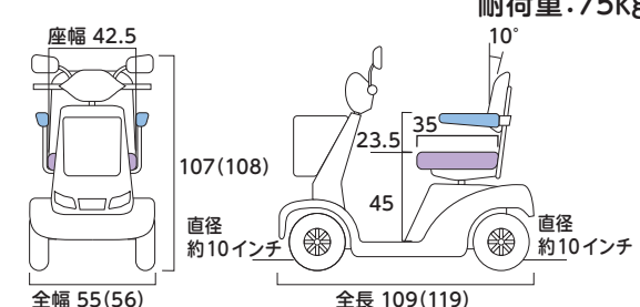
寸法図(単位:cm)
